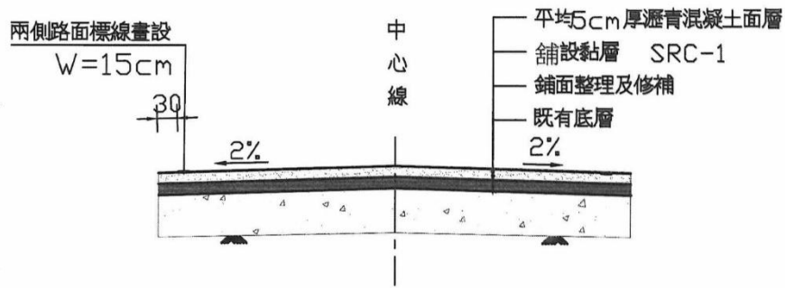
AC 路面標準斷面圖
