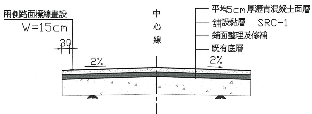
AC 路面標準斷面圖
